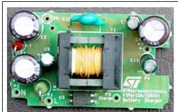
STEVAL-ISA020V1
